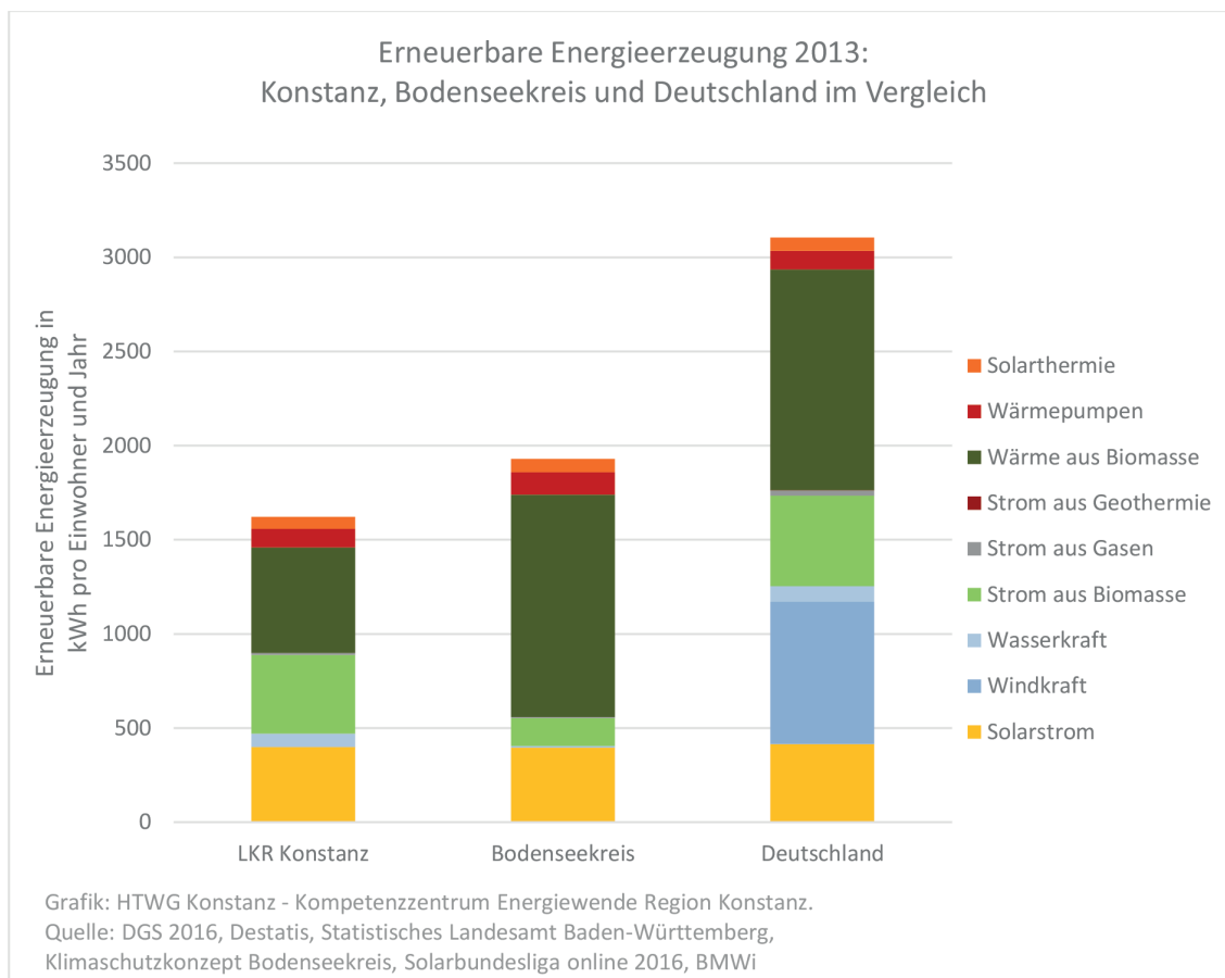
Abb. 19. Erneuerbare Energieerzeugung im Jahr 2013: Landkreis Konstanz, Bodenseekreis und Deutschland im Vergleich
