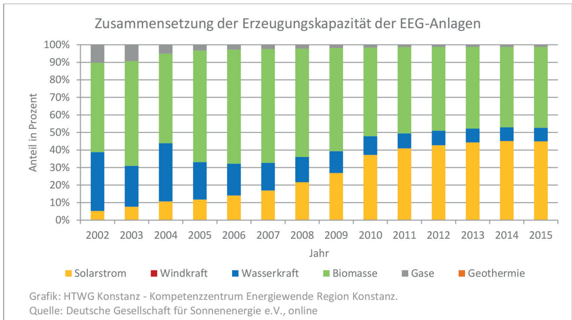
Abb. 24. Prozentuale Zusammensetzung der Erzeugungskapazität der EEG-Anlagen im Landkreis Konstanz
