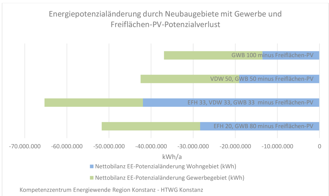
Abb. 165. Energiepotenzialänderung durch Neubaugebiete mit Gewerbe und Freiflächen-PV-Potenzialverlust
