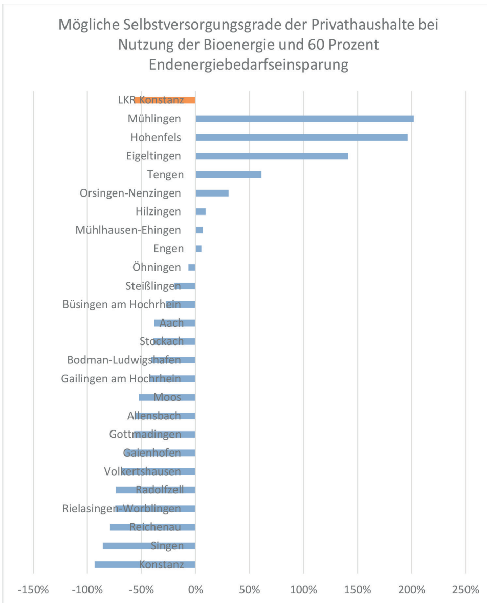
Abb. 150. Mögliche Selbstversorgungsgrade der Privathaushalte bei Nutzung der Bioenergie
