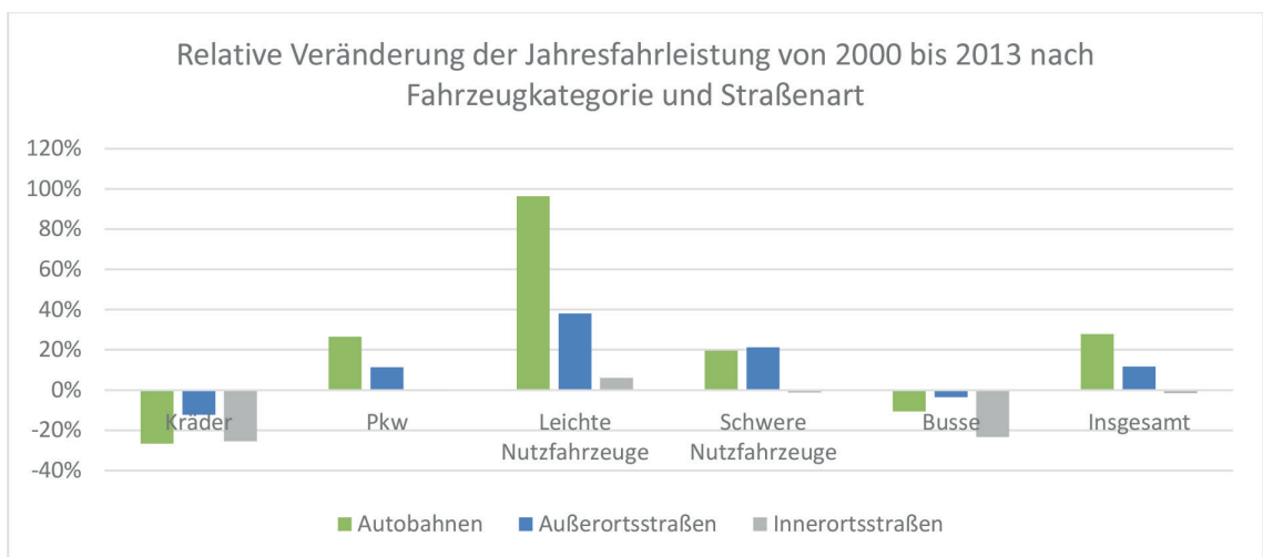
Abb. 42. Relative Veränderungen der Jahresfahrleistungen nach Straßenkategorien von 2000 bis 2013
