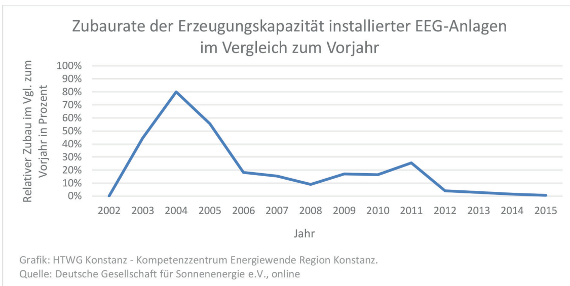
Abb. 22. Zubaurate der Erzeugungskapazität installierter EEG-Anlagen im Vergleich zum Vorjahr
