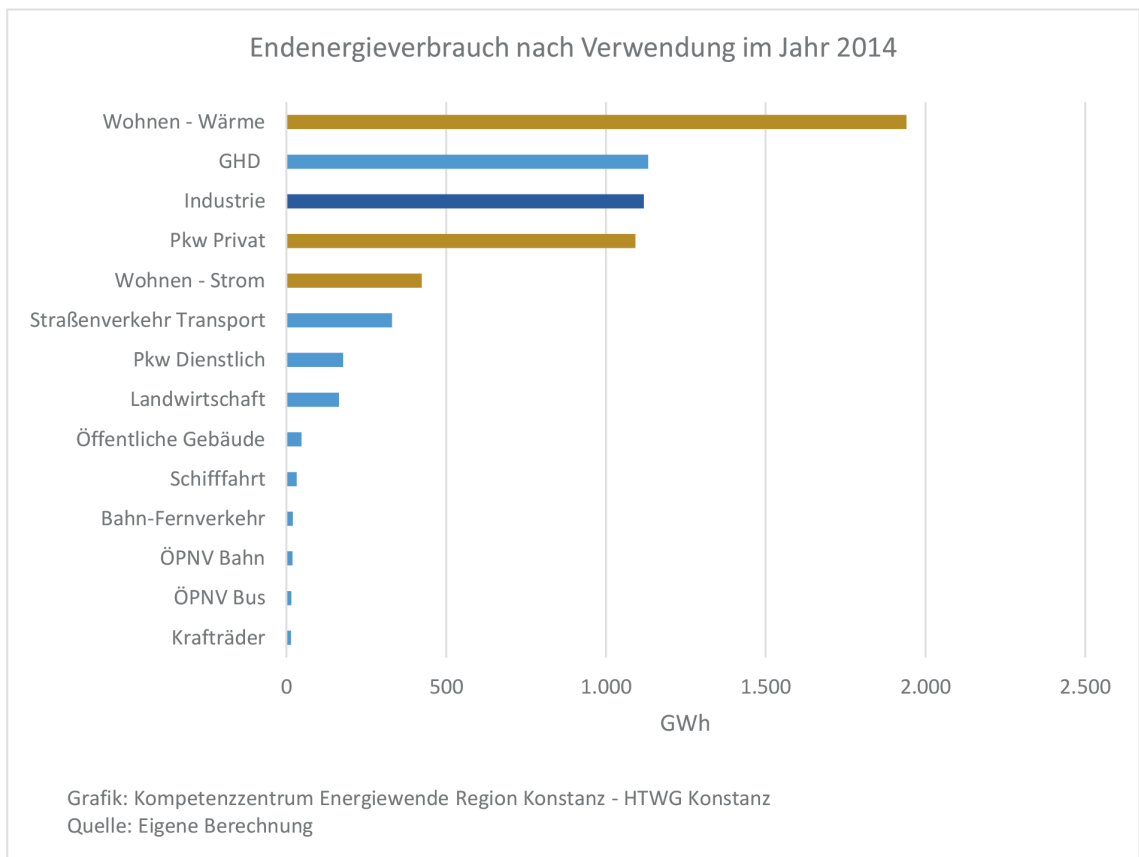
Abb. 16. Endenergieverbrauch nach Verwendung im Jahr 2014 in GWh
