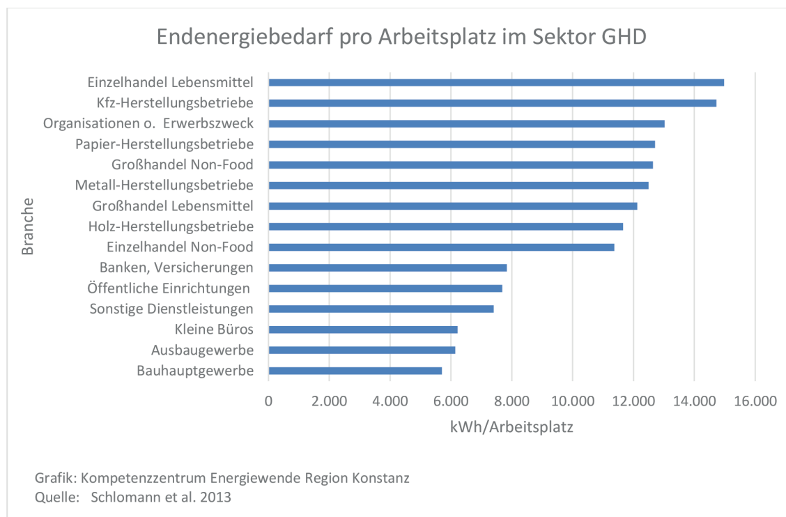
Abb. 110. Endenergiebedarf pro Arbeitsplatz im Sektor GHD
