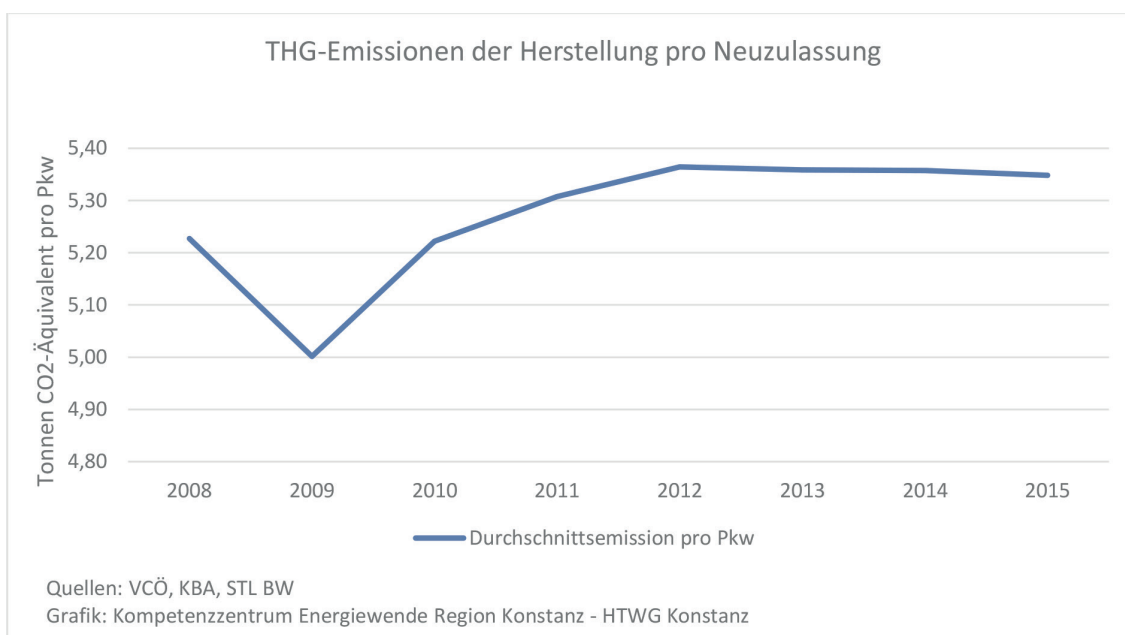
Abb. 69. THG-Emissionen der Herstellung pro Neuzulassung im Landkreis Konstanz
